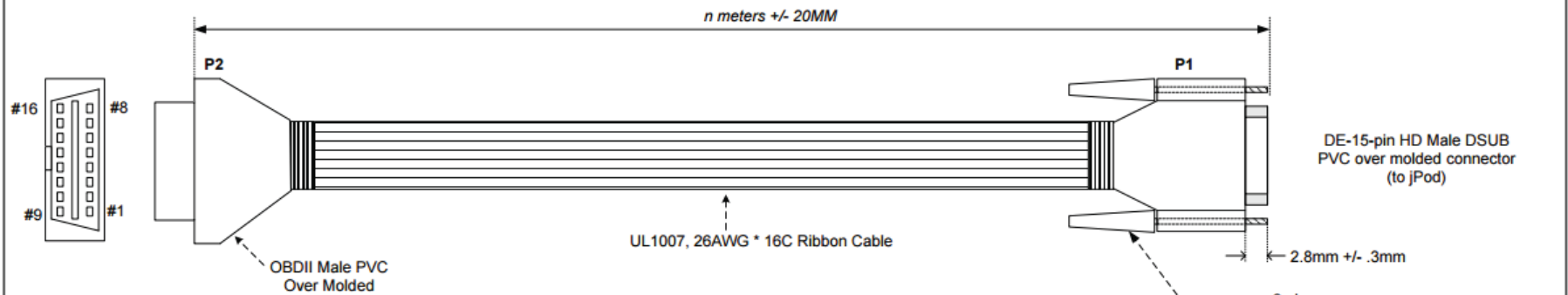
Wire Table
